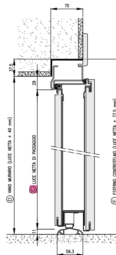
Configurazione con soglia tenuta aria-acqua-vento Configuration with air-water-wind tightness sill
