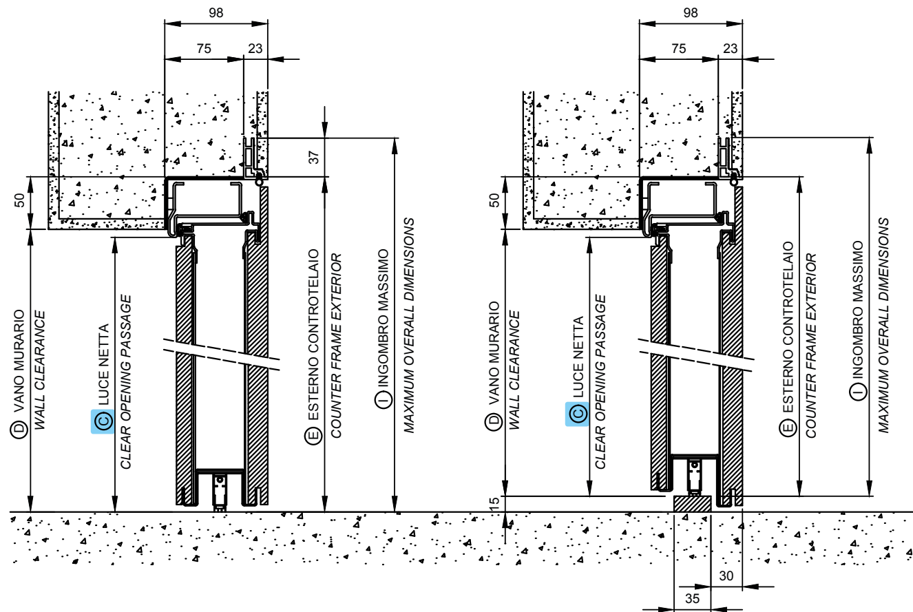
Configurazione pavimento complanare Flush floor configuration
